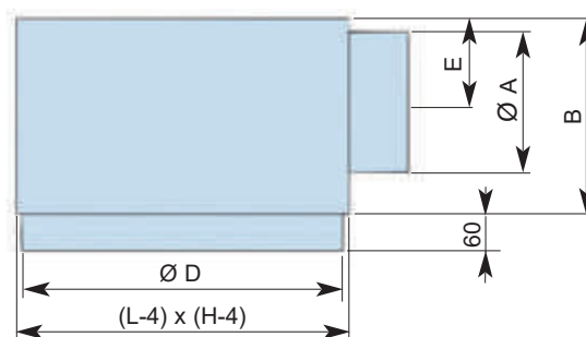
PLENUM PARA PLACA CIRCULAR
