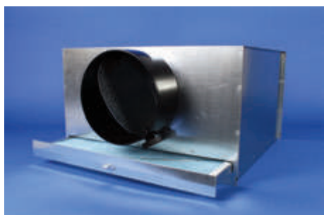
PLENUM+PORTAFILTRO (placa cuadrada)
