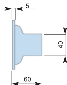
Mod. BIS con perfil conducto circular
