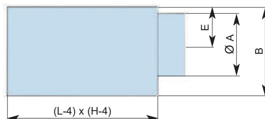
PLENUM PARA PLACA CUADRADA
