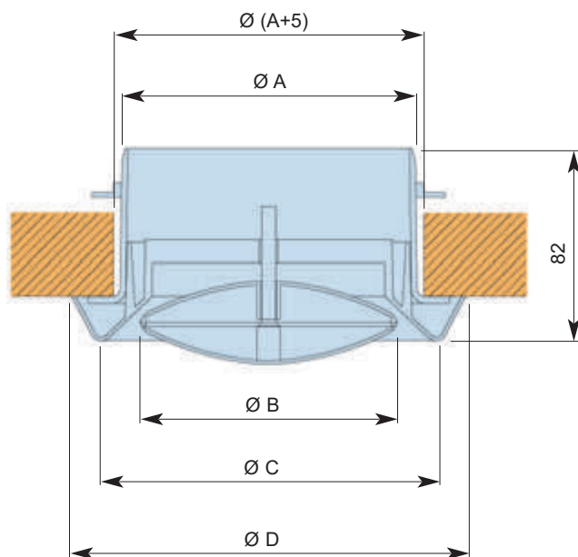
MODELO BCE Boca extractora.
