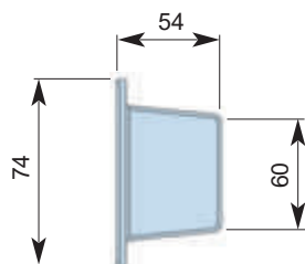
Mod. BIC con perfil conducto circular
